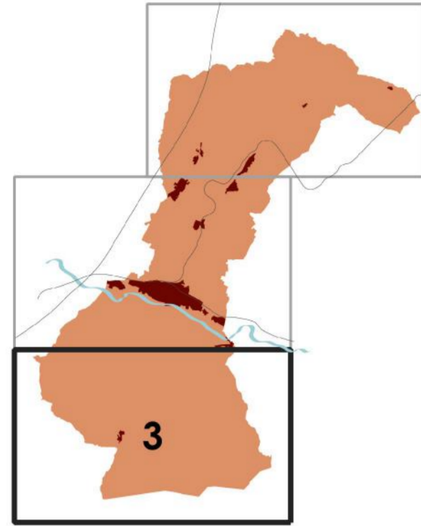
GEO08.3 - Carta della Microzonazione Sismica - FA0105
