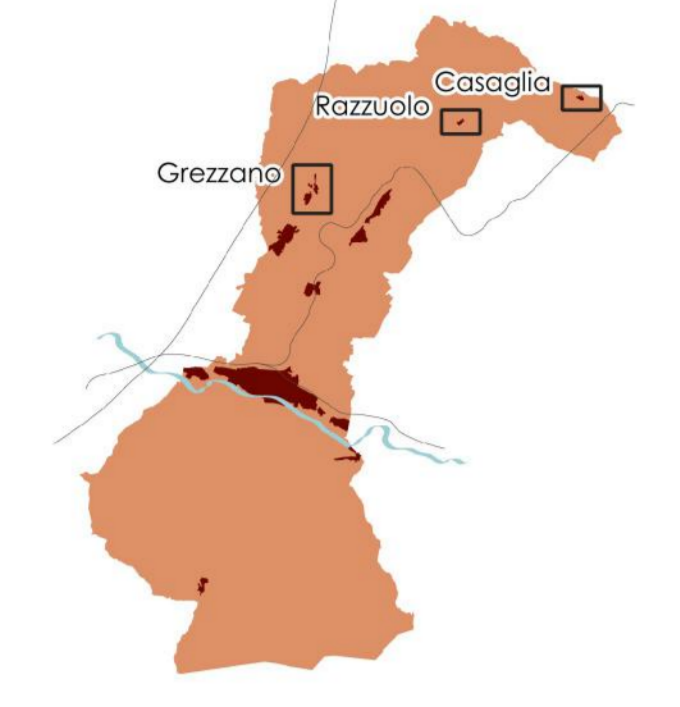
GEO04_a - Carta della esposizione sismica
